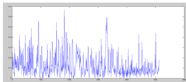
Figure 18. Coherence between ECG and EEG gamma wave (MIT BIH)
