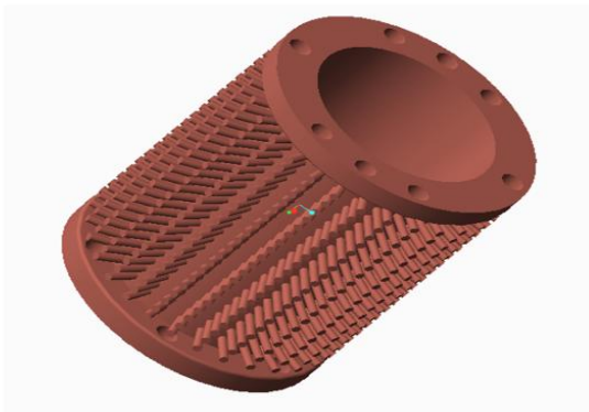
Fig2.4 cylindrical pin fins
