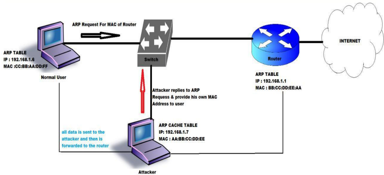
Fig. 2 ARP spoofing (MITM Attack)
