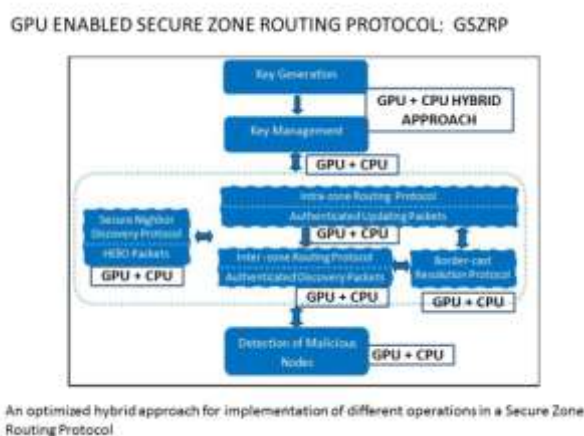
Fig. 2.CPU Vs. GPU
