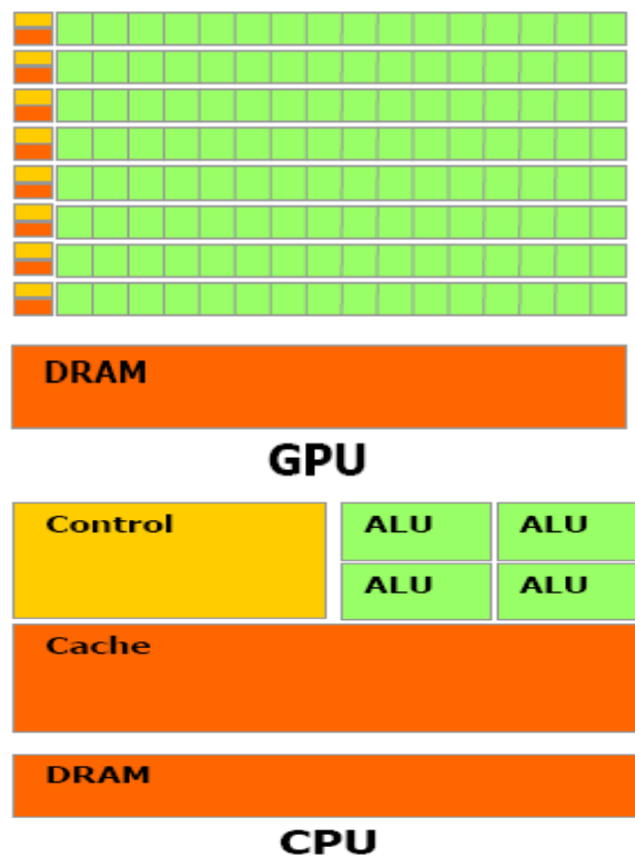
Fig. 1.CPU Vs. GPU
