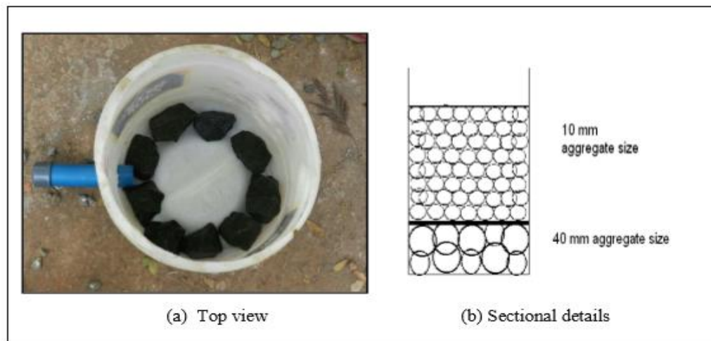
Fig. 3 : Trickling filter
