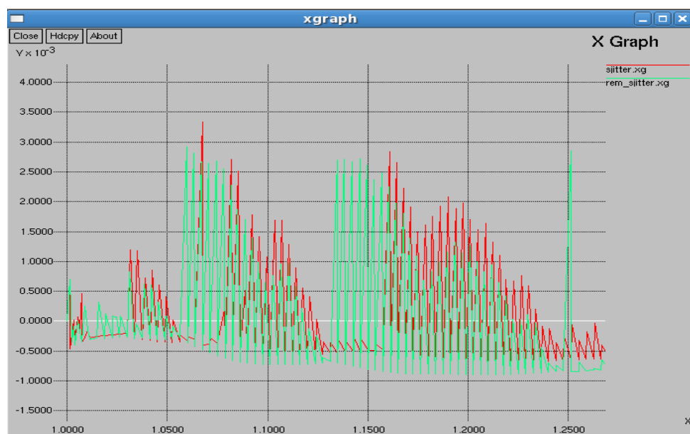
Fig 4: jitter
